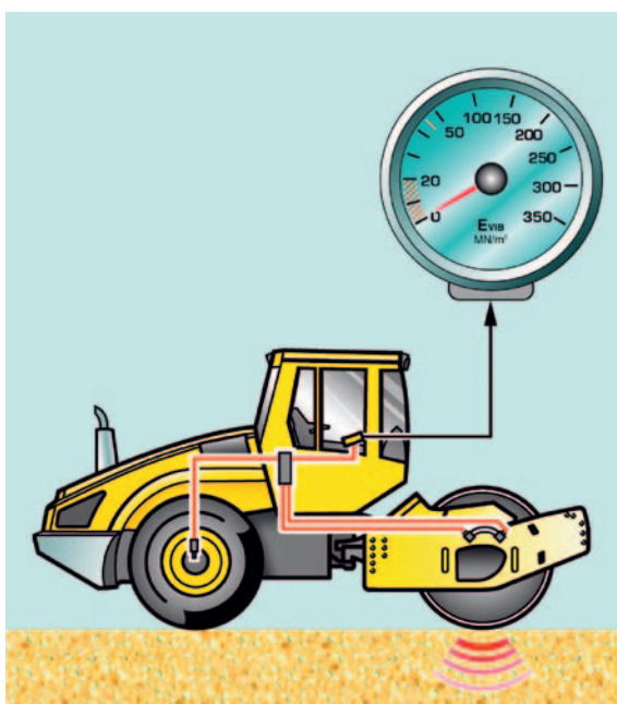
Der Einstieg: BOMAG E_{VIB} -Meter BEM.
