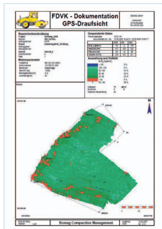
Präzise Verdichtungslandkarten mit BCM 05 positioning.
